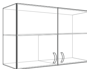
Шафа 100 В ш1000*г304*в570
