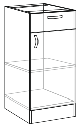
Стіл 40 НШ ш400*г464*в817
