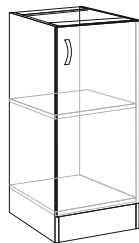
Стіл 30 Н ш300*г464*в817
