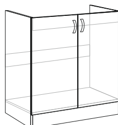
Стіл 80 НМ ш800*г464*в817
