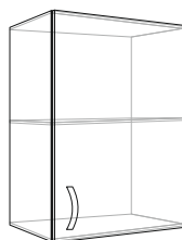
Шафа 40 В ш400*г304*в570
