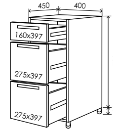
12 Низ 820*400 12/1 12/4 12/6
