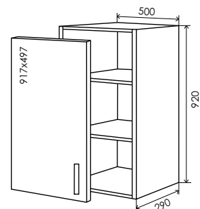
39 Верх 920*500 39/1
