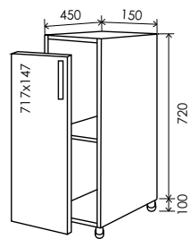
2 Низ 820*150 2/1
