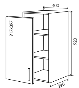
38 Верх 920*400 38/1
