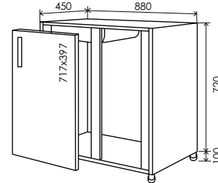
22 Низ мийка уні 820*880 22/1
