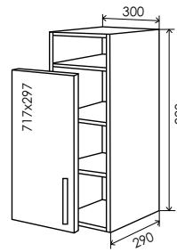
28 Верх 920*300 28/1
