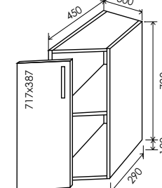
19 Низ 820*300 19/1
