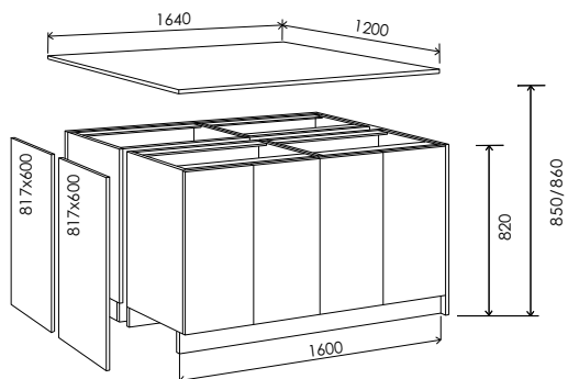
Острів 1 складається з 10 низ - 2шт.
