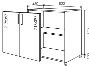
10 Низ 820*800 10/1
