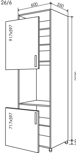
30 Пенал 2330*600 30/1
