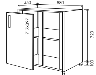
23 Низ уні 820*800 23/1
