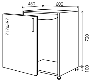
20 Низ мийка 820*600 20/1
