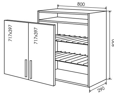
34 Верх сушарка 920*800 34/1
