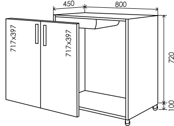
21 Низ мийка 820*800 21/1
