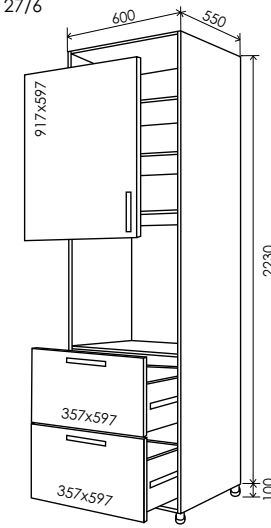
31 Пенал 2330*600 31/1 31/4 31/6
