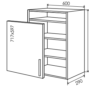
31 Верх 920*600 31/1
