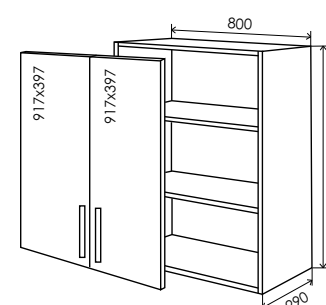
42 Верх 920*800 42/1
