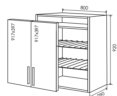
43 Верх сушарка 920*800 43/1
