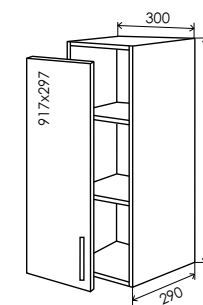
37 Верх 920*300 37/1
