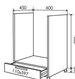
17 Низ духовка 820*600 17/1
