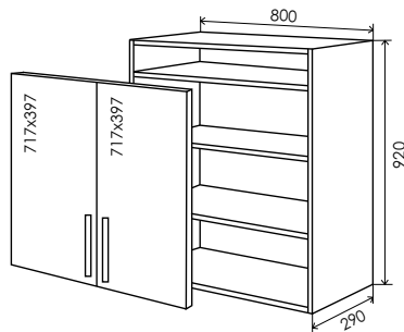
33 Верх 800*920 33/1
