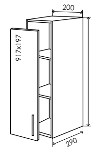
36 Верх 920*200 36/1
