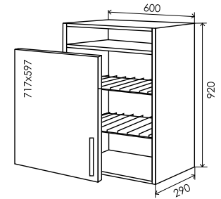
32 Верх сушарка 920*600 32/1
