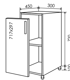
6 Низ 820*300 6/1 6/2
