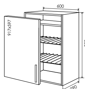
41 Верх сушарка 920*600 41/1
