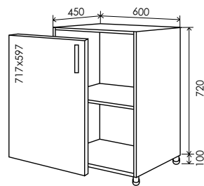
9 Низ 820*600 9/1
