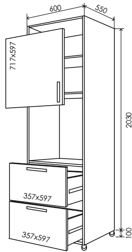
29 Пенал 2130*600 29/1 29/4 29/6
