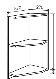
18 Низ консоль 820*290
