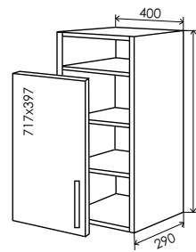
29 Верх 920*400 29/1
