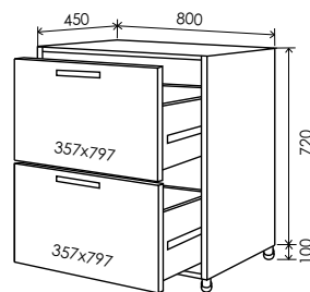
16 Низ 820*800 16/1 16/4 16/6
