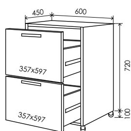
15 Низ 820*600 15/1 15/4 15/6
