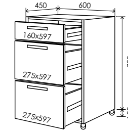
13 Низ 820*600 13/1 13/4 13/6
