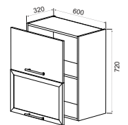
Верх 2Д МДФ+АГТ 600_320_720 (GW60) H-720mm., W-600mm.
