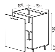
Низ 1Д 600_500_720 (D60) H-720mm., W-600mm.
