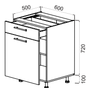
Низ 1Ш 1Д 600_500_720 (D601S) H-720mm., W-600mm.
