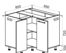
Низ угол 850_850_500_720 (A1) H-720mm., W-850mm.
