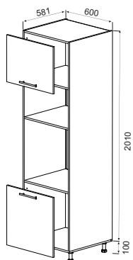
Пенал 2Д 600-600-2010 (D60COL) H-720mm., W-600mm.
