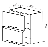
Верх 2Д МДФ+АГТ 800_320_720 (GW80) H-720mm., W-800mm.
