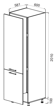
Пенал 2Д под холодильник 600-600-2010 (D60FRIDGE) H-720mm., W-600mm.
