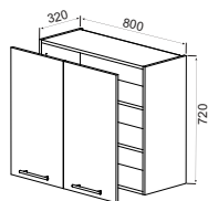
Верх 2Д 800_320_720 (G80) H-720mm., W-800mm.
