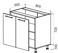
Низ 2Д 800_500_720 (D80) H-720mm., W-800mm.
