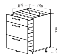
Низ 3Ш 600_500_720 (D603S) H-720mm., W-600mm.
