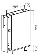
Низ 1Д 150_500_720 (D15) H-720mm., W-150mm.
