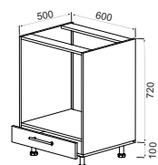
Низ духовка 600_500_720 (D60P) H-720mm., W-600mm.
