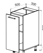
Низ 1Д 300_500_720 (D30) H-720mm., W-300mm.
