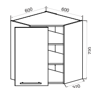
Верх угол 600_600_720 (A4) H-720mm., W-600mm.
