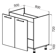
Низ 2Д 800_500_720 (DZ80) H-720mm., W-800mm.
