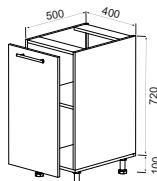
Низ 1Д 400_500_720 (D40) H-720mm., W-400mm.
