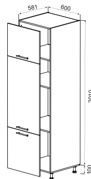
Пенал 3Д 600-600-2010 (D60COL MID) H-720mm., W-600mm.
